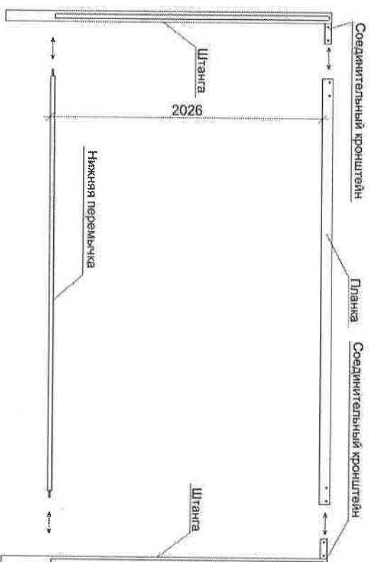
Схема сборки минифутбольных ворот
